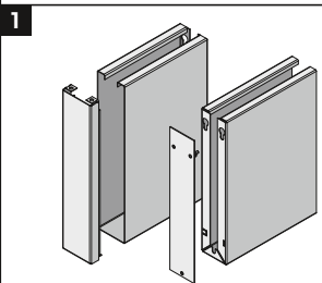
1 Endkappe / Stirndeckel mit F-Lippe End cap / end cover with F-flap Capuchon d'extrémité / cache lateral avec F
